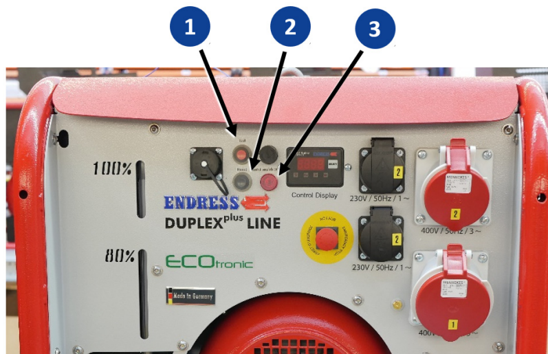
Abb. 8-3 Isolationsüberwachung
