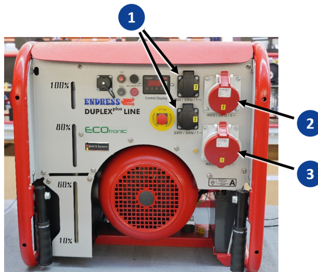
Abb. 7-4 Verbrauchsmittel anschließen
